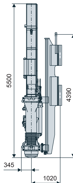
DELMAG Dieselpär diesel pile hammer D19-52
